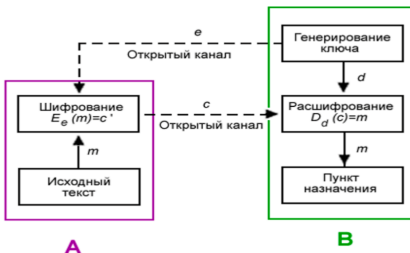
Рисунок 1. Ассиметричная схема шифрования
