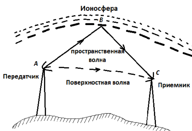
Рисунок 2. Распространение волн в атмосфере
