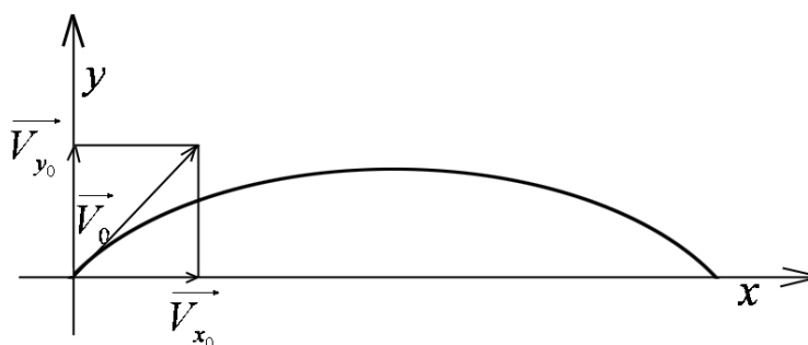
Рисунок 1. Траектория полета снаряда
