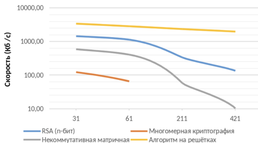
Рисунок 2. Зависимость скорости шифрования от длины ключей
